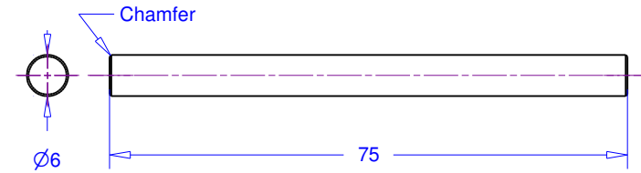
Stop Bar (1off M.S.)
